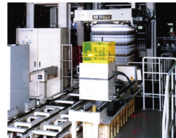
バルクデパレタイザー(低床式・高床式)
