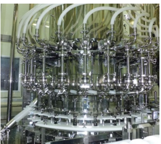
充填キャッパー
