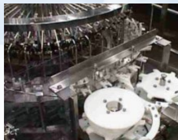
RBS型リンサー(ロータリー式)
